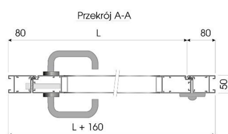
Detal połączeń okna, maskownicy i skrzydła Zlicowanie elementów skrzydła drzwi
