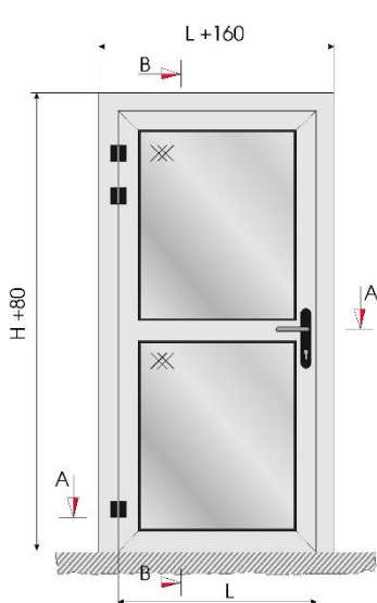
Współpłaszczyznowość ościeżnicy i skrzydła drzwi
